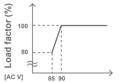
2.5.3 UUHP150 | 入力ディレーティング曲線
