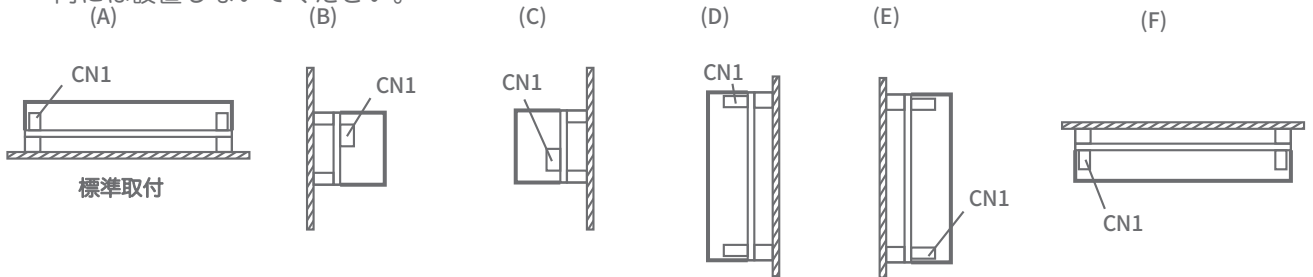
2.4.1 標準取付
