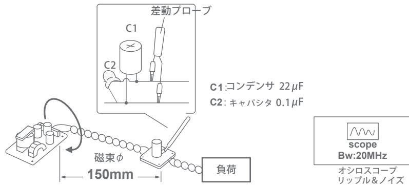
1.5.1 UUHP150 | 出力リップル&ノイズの測定例
