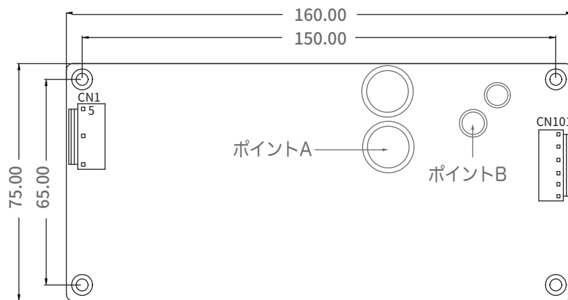
A点およびB点は温度測定の測定ポイントです。
