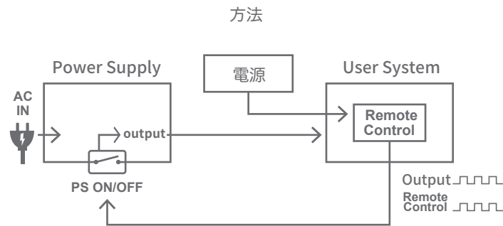
3.2.1 リモートON/OFF回路の使用例
