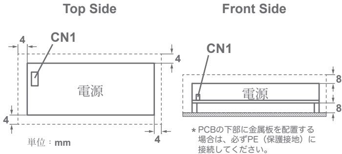
2.1.1 UUHP | オープンフレームの設置距離
