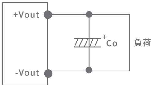
3.4.1 外部コンデンサを接続する例
