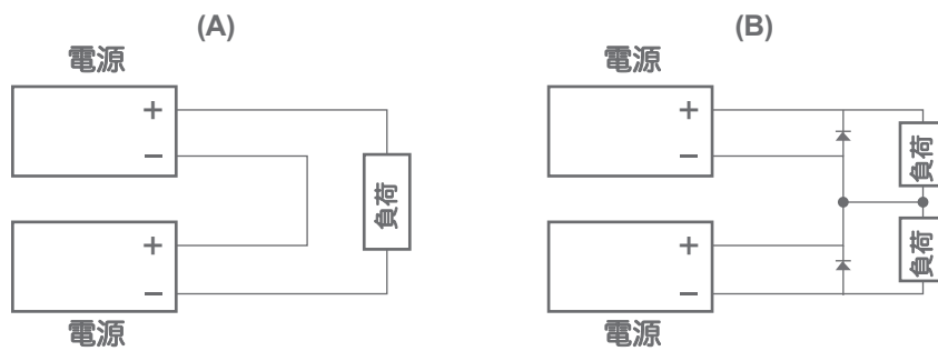
3.3.1 直列運転時の接続例
