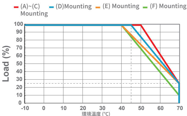
2.5.2 UUHP150 | 取り付け方向別出力ディレーティング曲線
