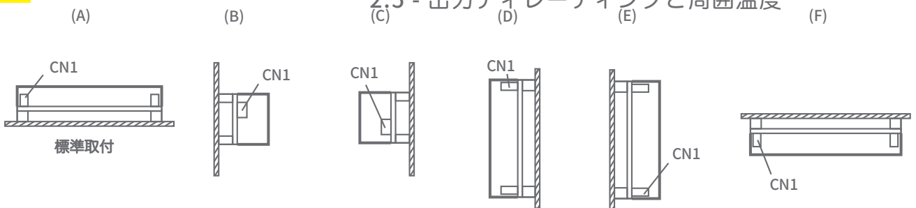
2.5.1 取付方向
