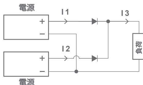
3.3.2 冗長運転時の接続例
